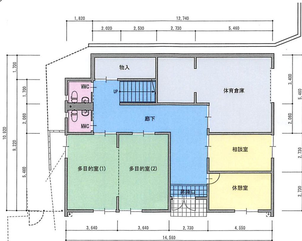
1階平面図
